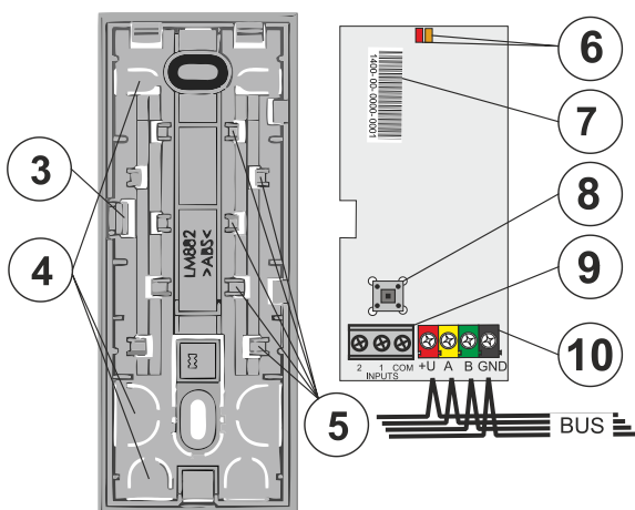
Rysunek 2: 3 – zatrzask płytki PCB; 4 – otwory na przewody; 5 – zaczepek do mocowania przewodów; 6 – czerwona i żółta dioda LED; 7 – numer seryjny; 8 – sabotaż; 9 – złącze czujki magnetycznej; 10 – wejście magistrali;
